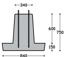
vooraanzicht
