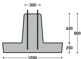
vooraanzicht
