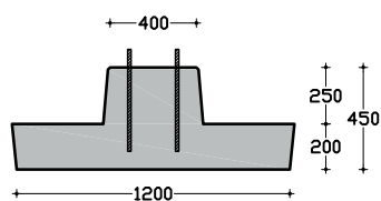
vooraanzicht
